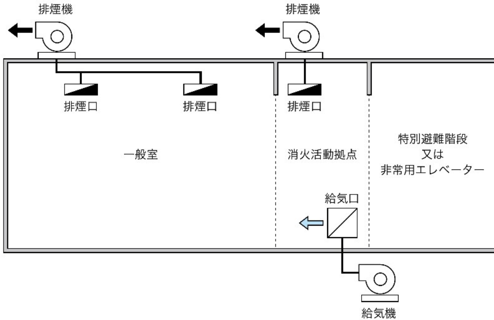
（排煙設備の構成例）
