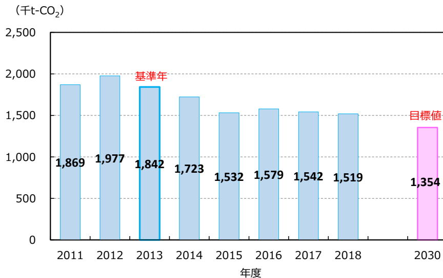
図 2-11 市内の温室効果ガス排出量の推移
