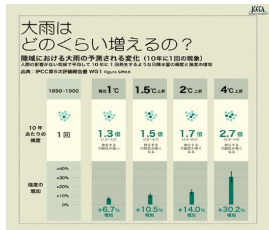
図 2-8 気温上昇による大雨の増加予測 出典)IPCC 第6次報告書 JCCCAウェブサイト
