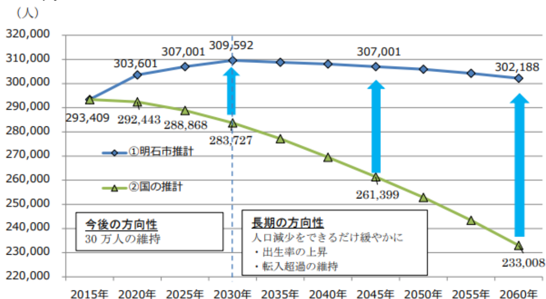
図 2-3 人口の推移と将来推計
