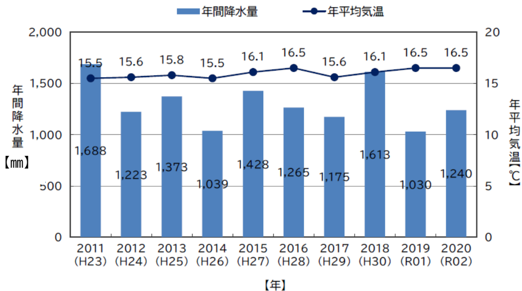
図 2-2 年平均気温と年間降水量の推移
