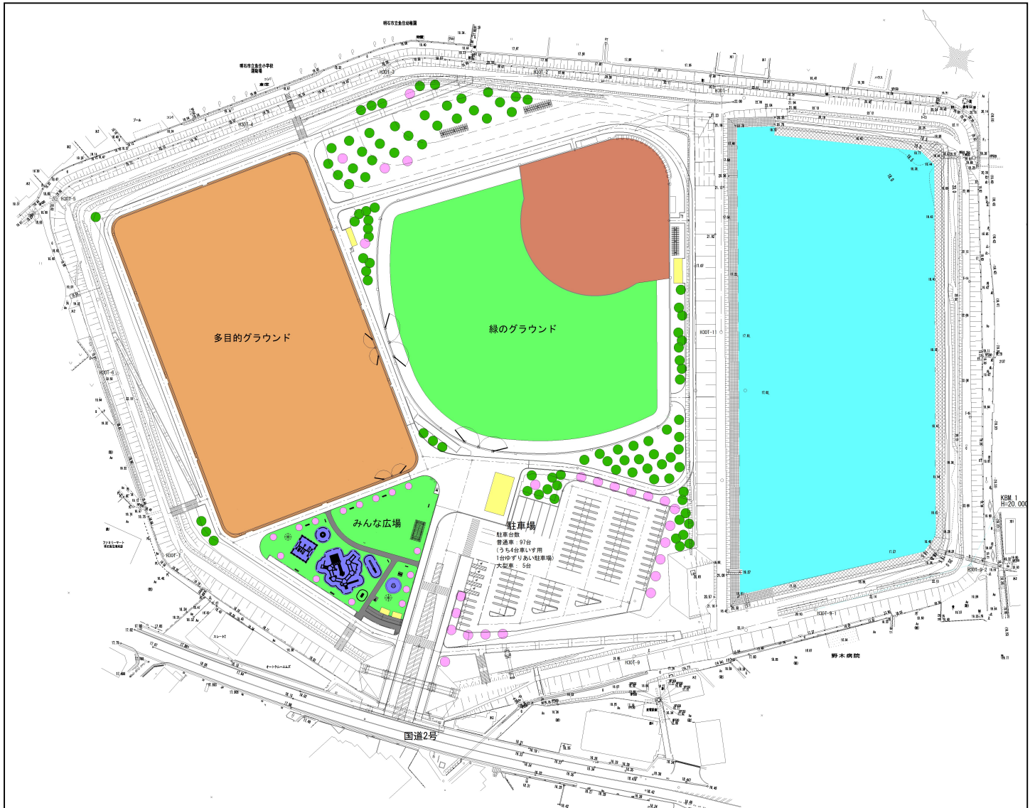
1 7号池魚住みんな公園 全体平面図
