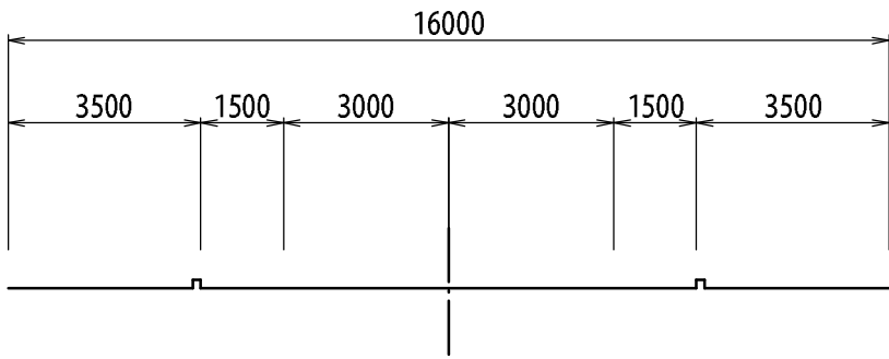
C-C断面 山手環状線
