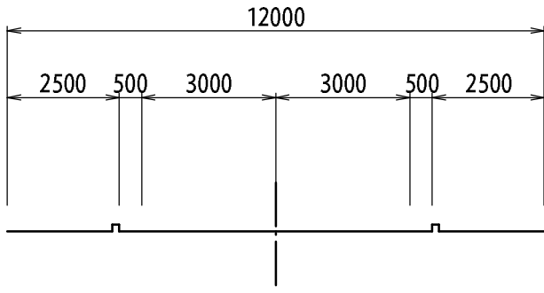
A-A断面 大久保石ヶ谷線
