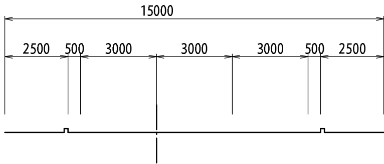
E-E断面 大久保石ヶ谷線
