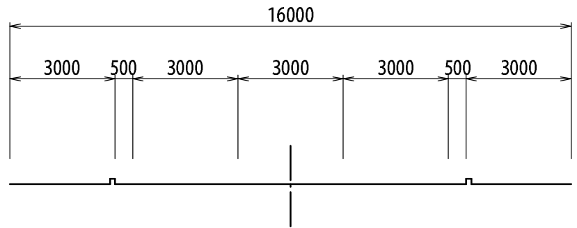
F-F断面 山手環状線
